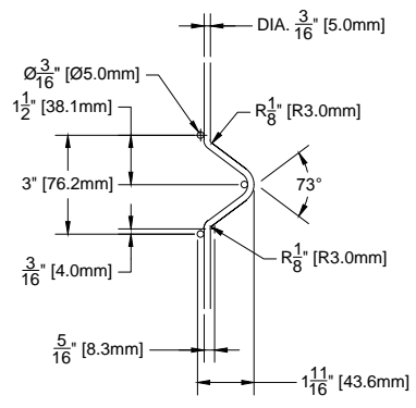
1 RIB DETAIL SCALE: NTS
