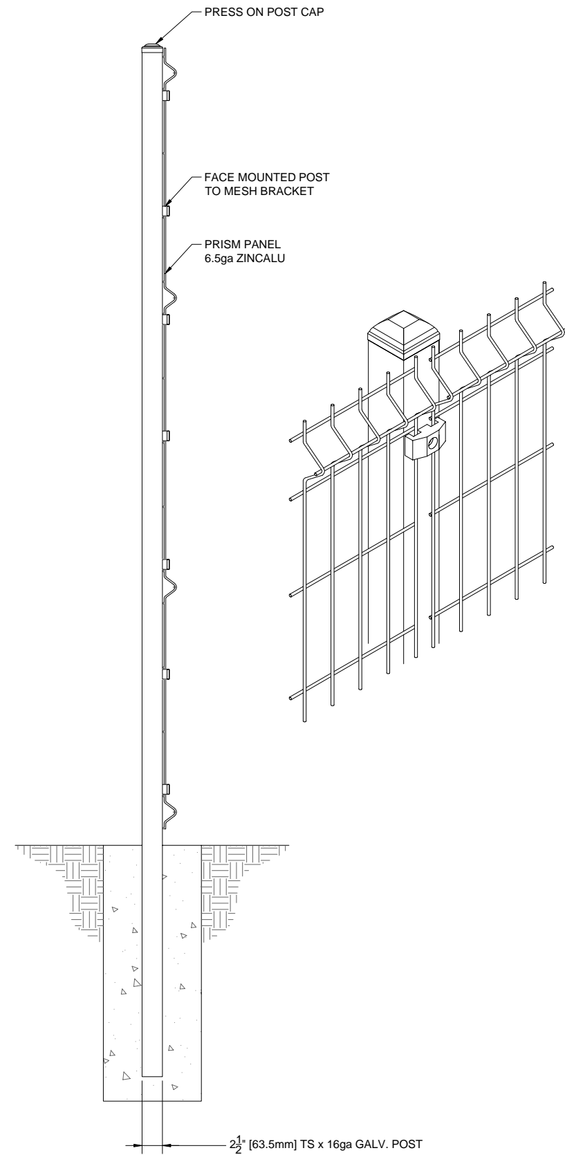
A 8'W x 8'H PANEL SECTION SCALE: NTS
