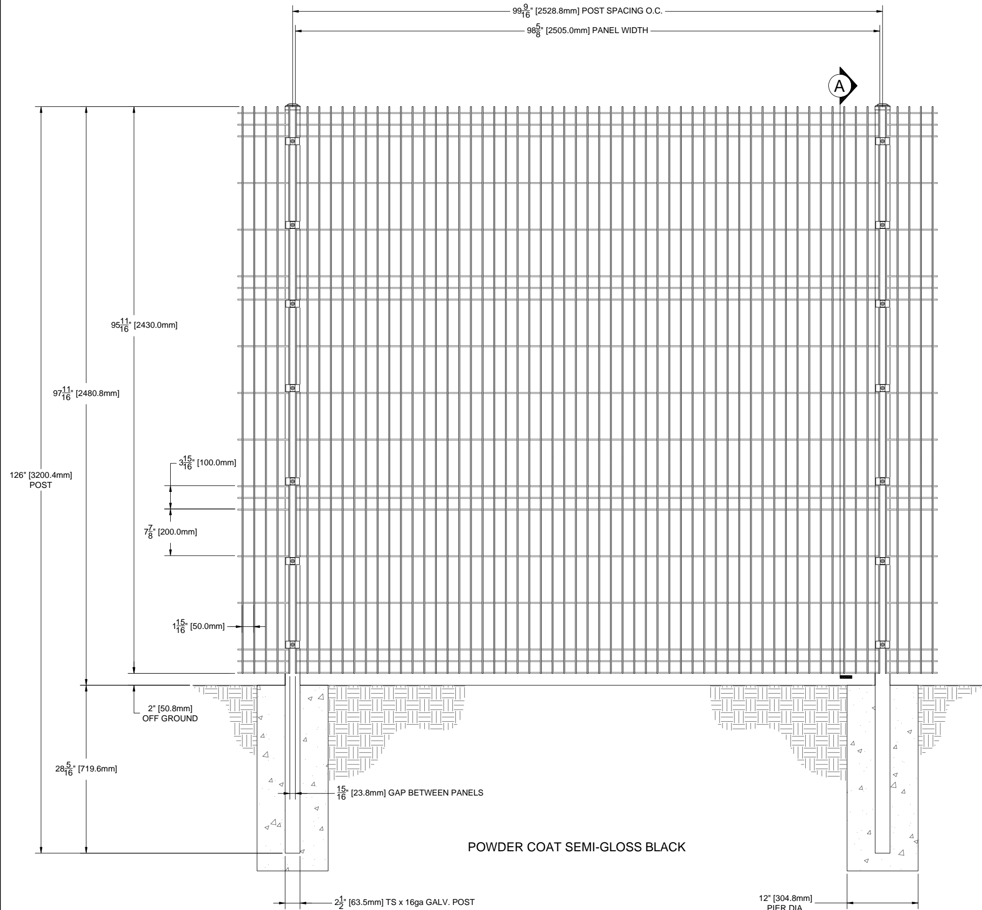
1 8'W x 8'H PANEL ELEVATION SCALE: NTS
