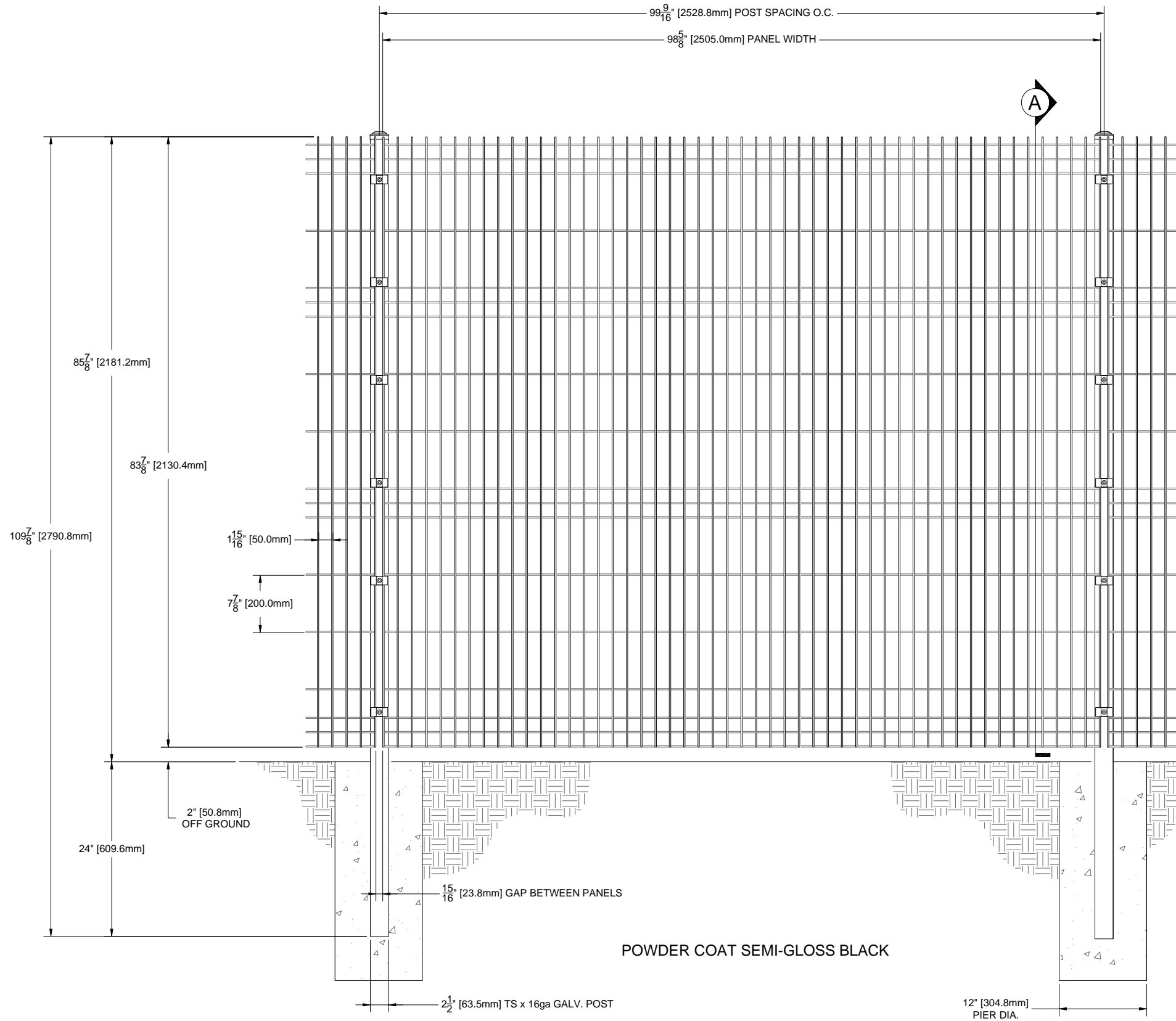
1 8'W x 7'H PANEL ELEVATION SCALE: NTS
