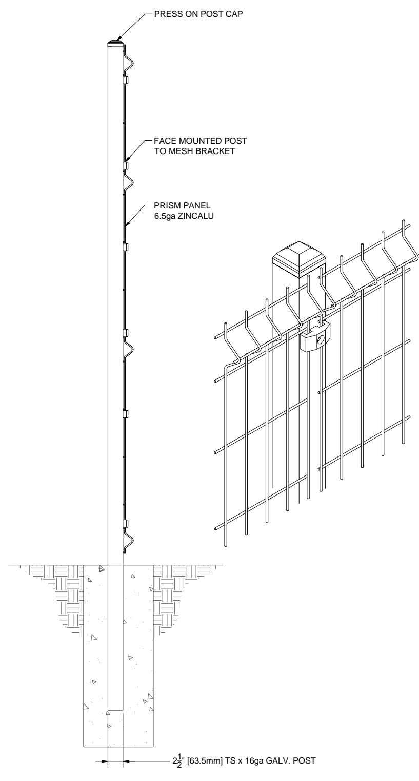
A 8'W x 7'H PANEL SECTION SCALE: NTS
