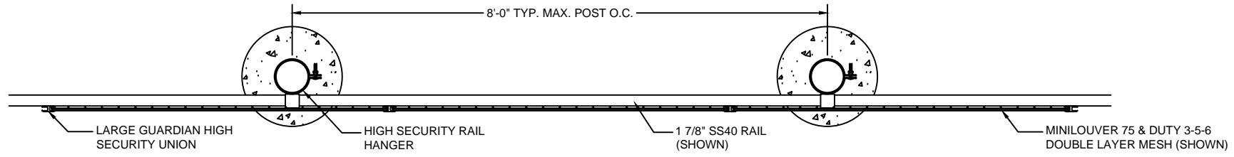
2 GUARDIAN 7000-GL PLAN SCALE: NTS
